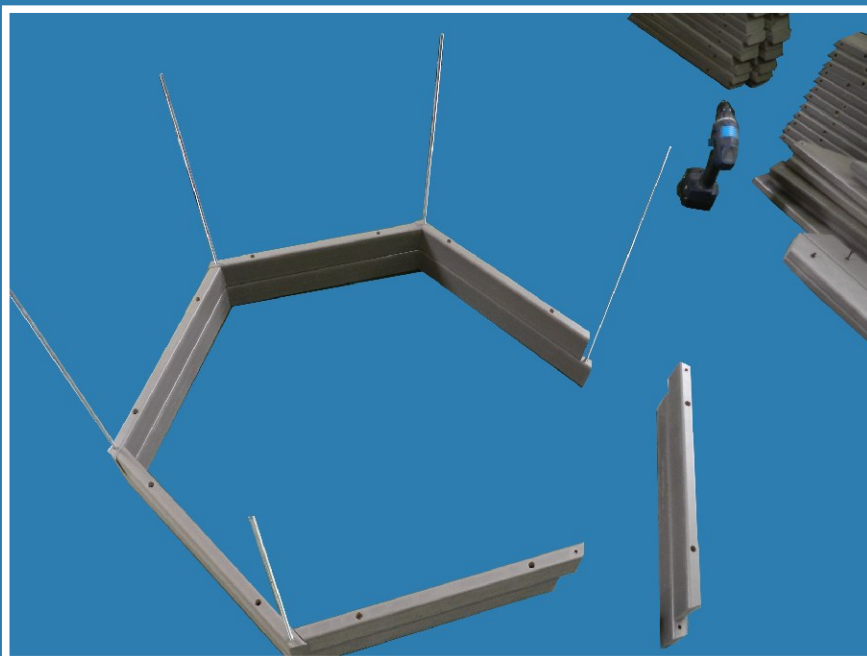
05 Składanie ścian donicy etap 2
